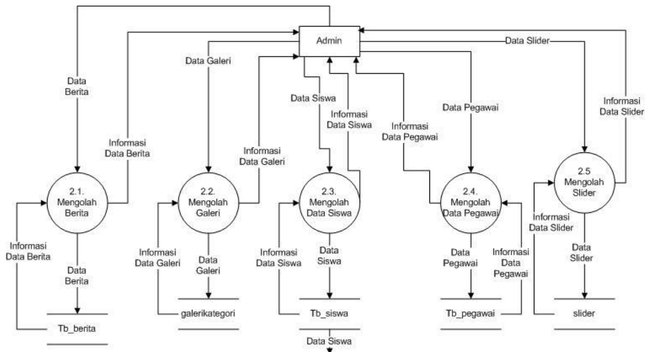
Gambar 3.4 DFD Level 2 Proses Mengolah Data
