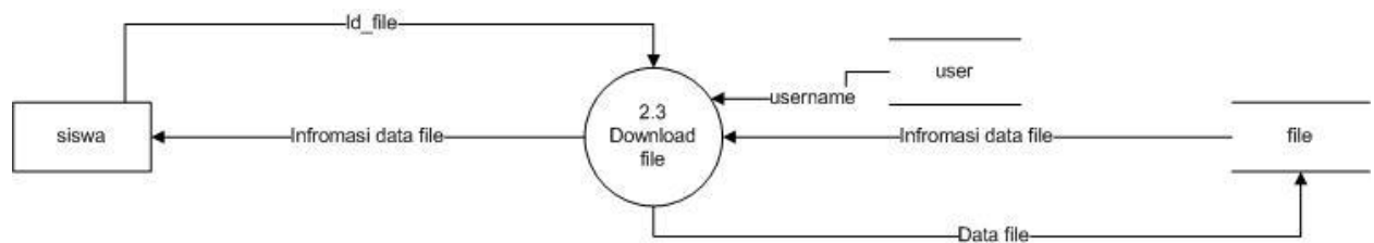
Gambar 3.14 DFD Level 2 Proses Mengolah Data Siswa
