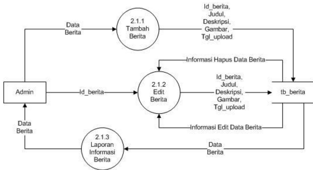
Gambar 3.5 DFD Level 3 Pengelolaan Berita
