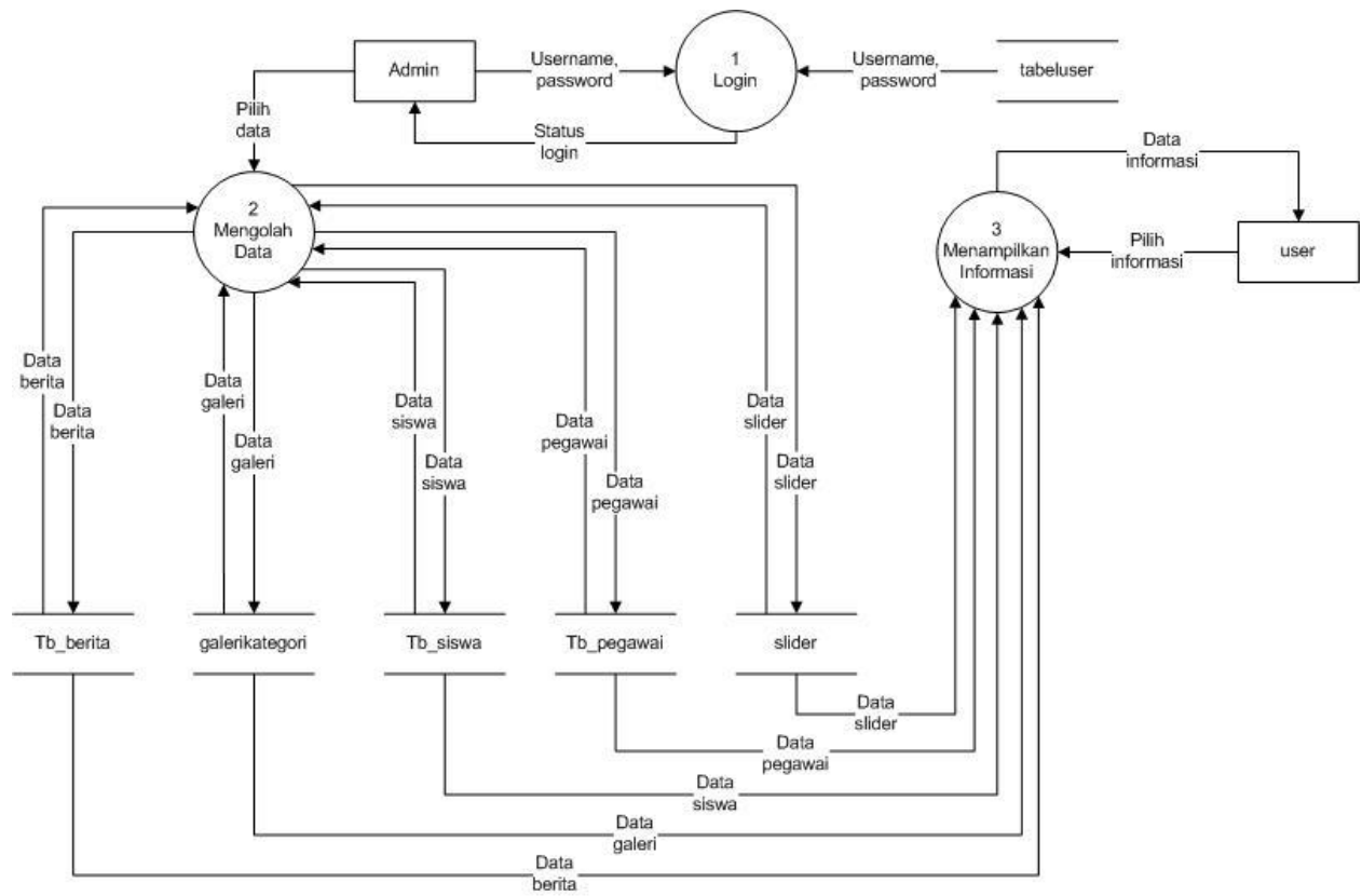
Gambar 3.2 DFD level 1 Web Profil SMA Negeri 1 Sumberlawang
