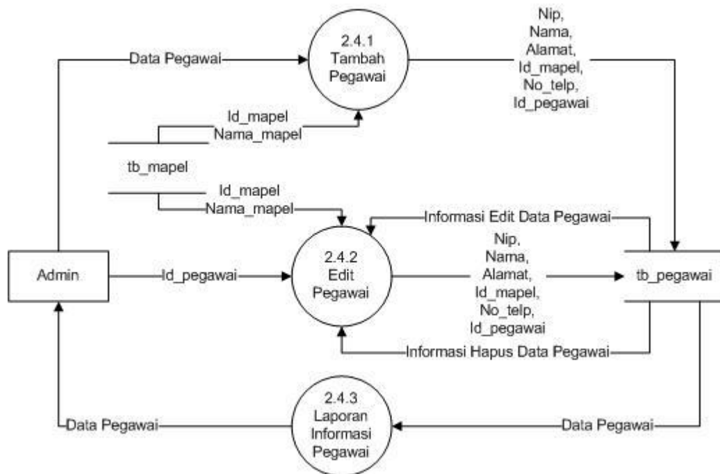
Gambar 3.8 DFD Level 3 Pengelolaan Data Pegawai
