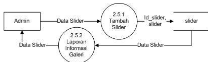
Gambar 3.9 DFD Level 3 Pengelolaan Slider
