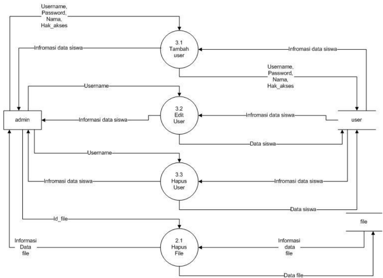
Gambar 3.12 DFD Level 2 Proses Mengolah Data Admin
