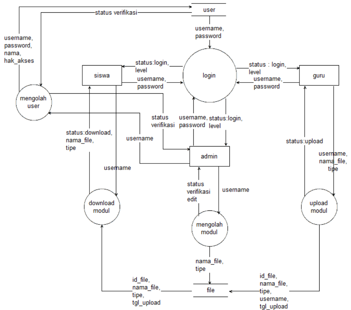
Gambar 3.11 DFD Level 1 E-learning SMA Negeri 1
