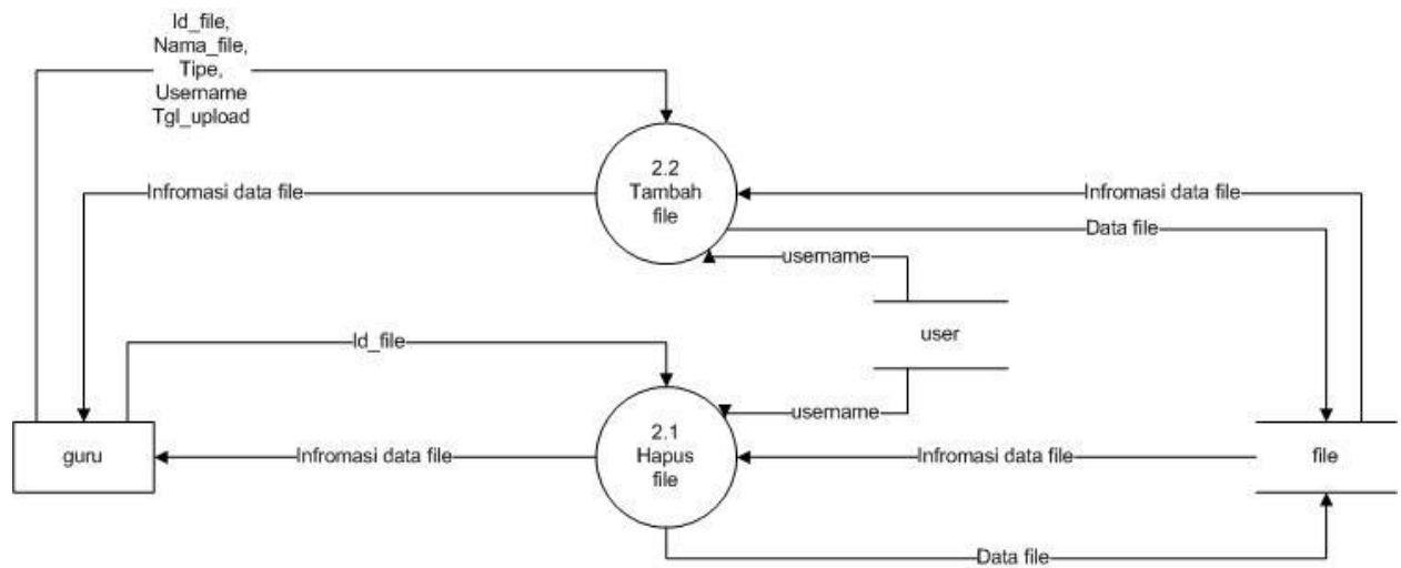
Gambar 3.13 DFD Level 2 Proses Mengolah Data Guru
