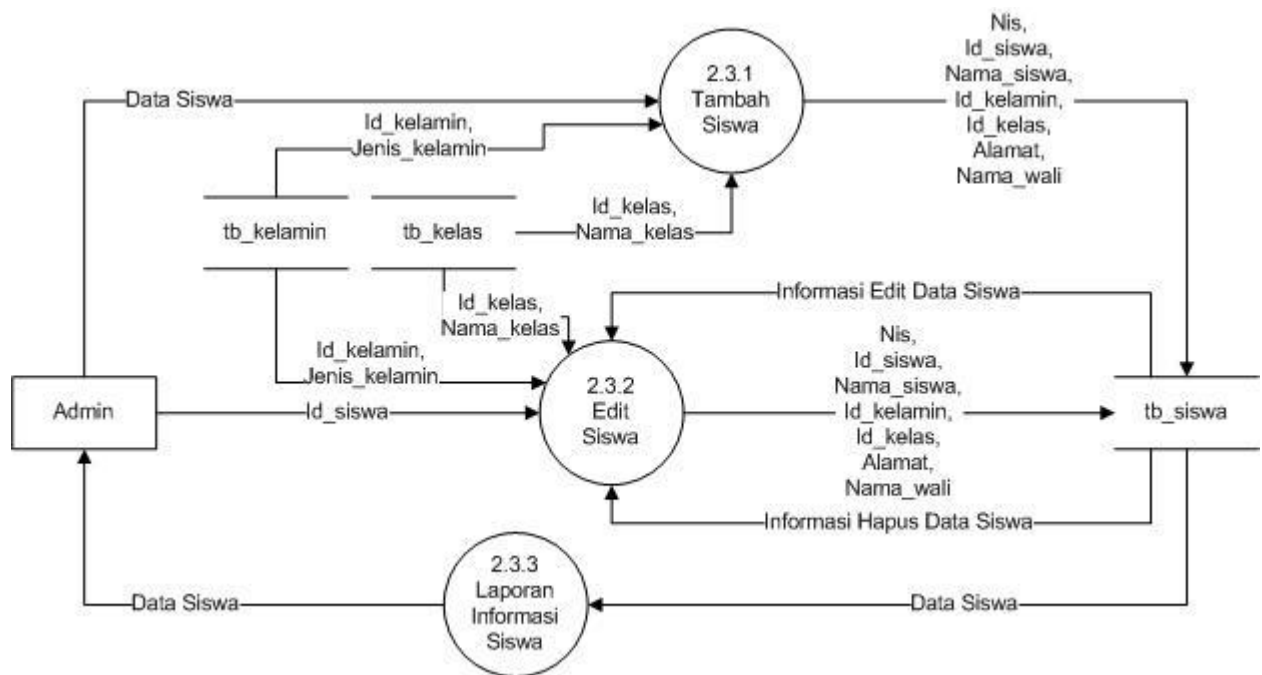
Gambar 3.7 DFD Level 3 Pengelolaan Data Siswa
