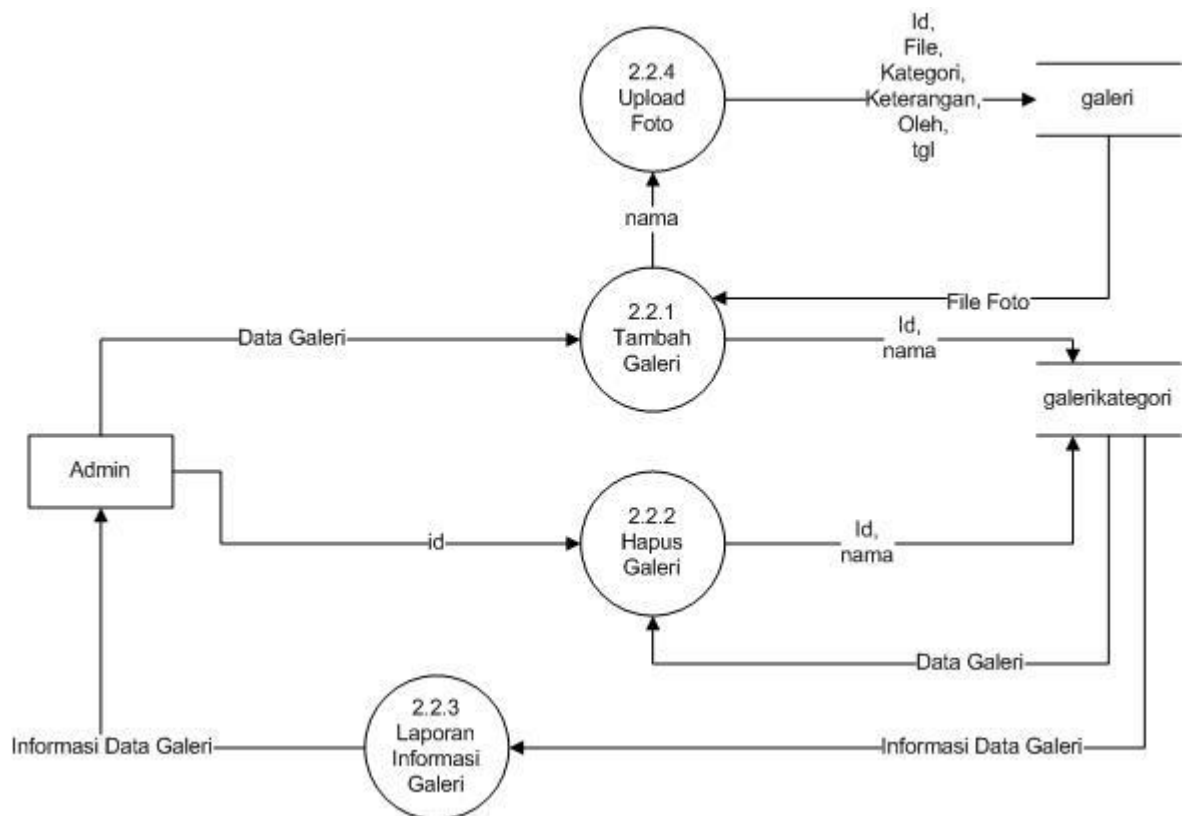
Gambar 3.6 DFD Level 3 Pengelolaan Galeri
